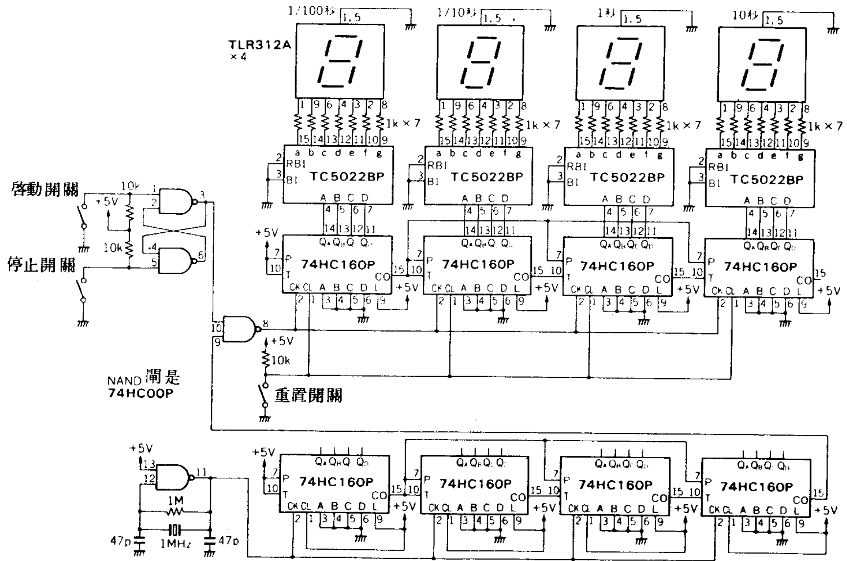
碼錶的電路圖 (能計數到 99.99 秒)
