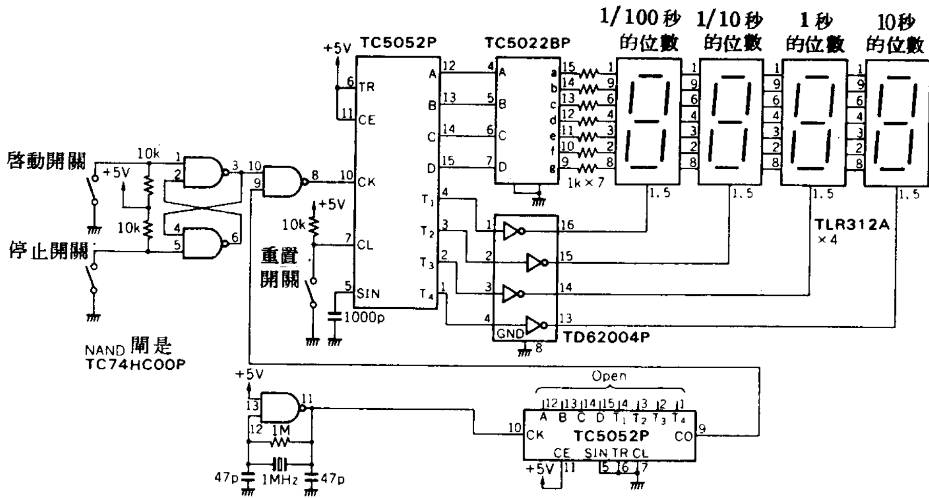
碼錶的電路圖(使用計數器專用IC)
